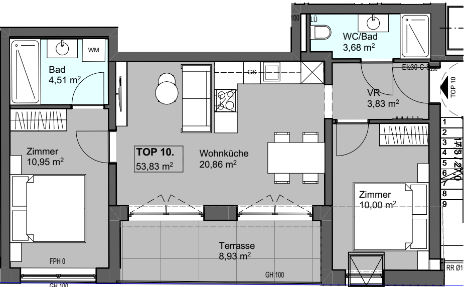
Variante 3 Zimmer
